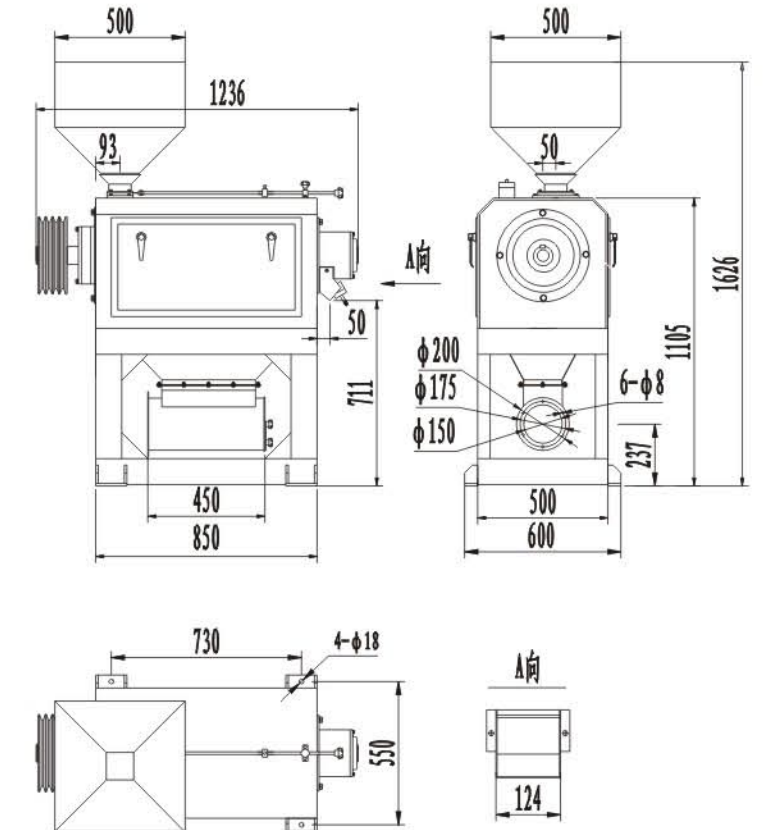
(外形尺寸与地脚安装图)
